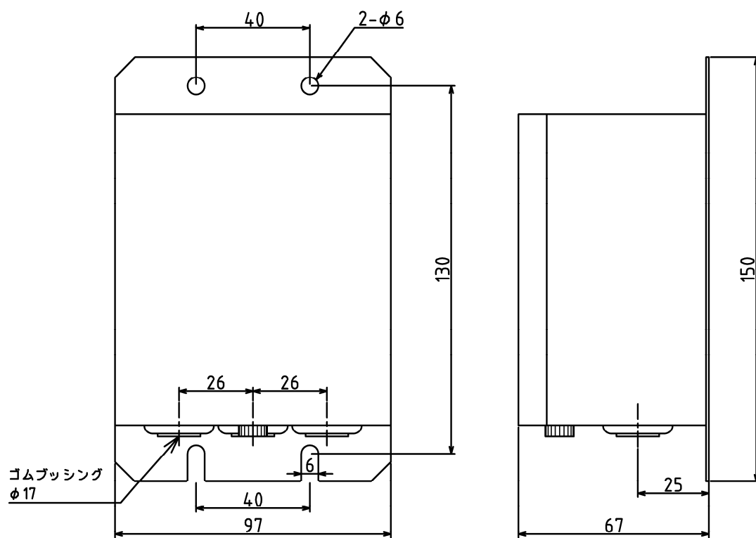
型番：TSS-A1SA-025 外形寸法図
