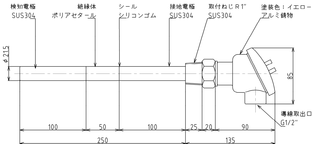
型番：TSS-A1SA-025 外形寸法図
