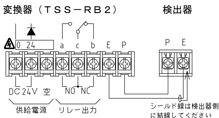
端子配列及び結線図
