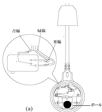
フロート垂直時
