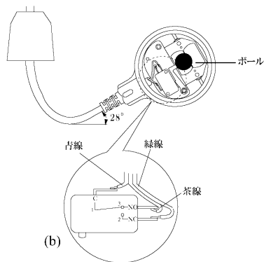
フロート上昇時
